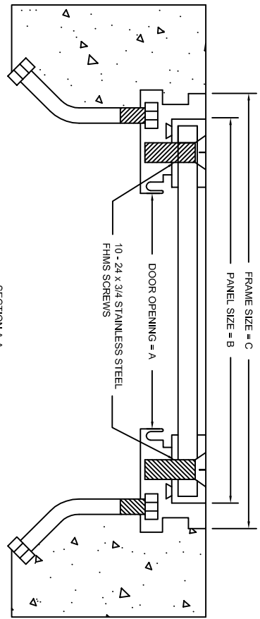
SECTION A-A
