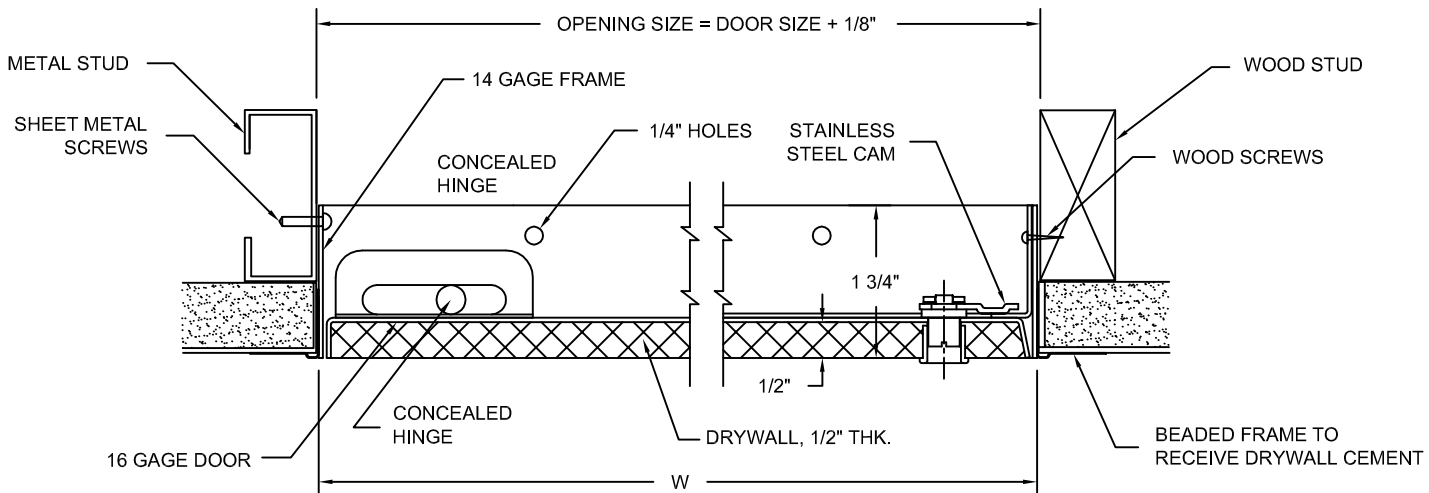
SECTION A-A
