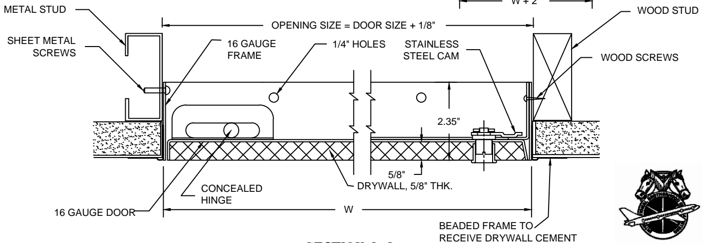
SECTION A-A
